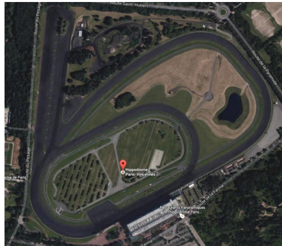
Rysunek 1. Zdjęcie satelitarne hipodromu
