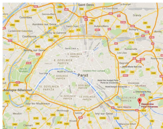
Rysunek 2. Lokalizacja toru w Paryżu
